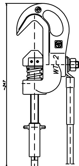
Zacisk fazowy WT-2/A (do szyn płaskich i przewodów okrągłych - do zamocowania w głowicy drążka UDI) Wykonanie „A”
