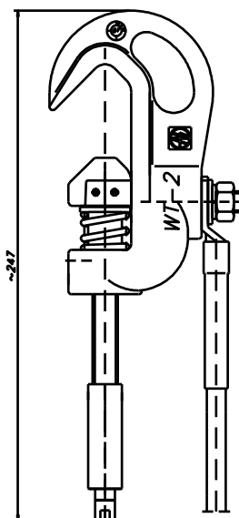
Zacisk fazowy WT-2/B (do szyn płaskich i przewodów okrągłych - do zamocowania w zatrzasku głowicy drążka UDI) Wykonanie „B”
