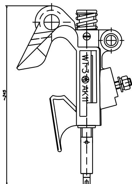
Zacisk fazowy WT-3/B (do zamocowania w zatrasku główicy drążka UDI) Wykonanie „B”
