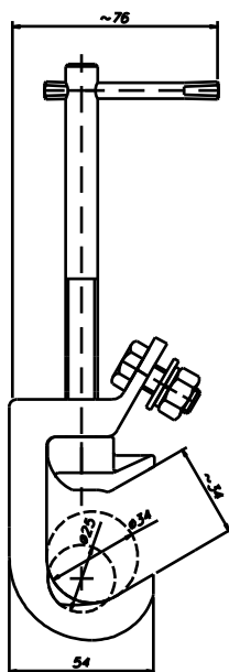
Zacisk uziomowy WR-K25 (do szyn płaskich, przewodów okrągłych i do przyłącza typu kula)
