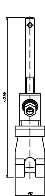
Zacisk uziomowy WR-K25 (do szyn płaskich, przewodów okrągłych i do przyłącza typu kula)
